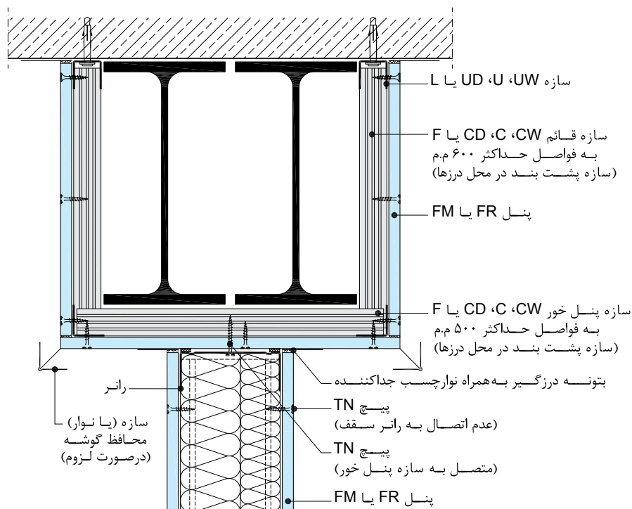
اتصال دیوار خشک به پوشش محافظ تیر (ثابت)
