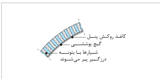
پوشش کاری تک لایه
