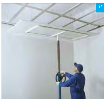
استقرار پل با استفاده از بالابر
