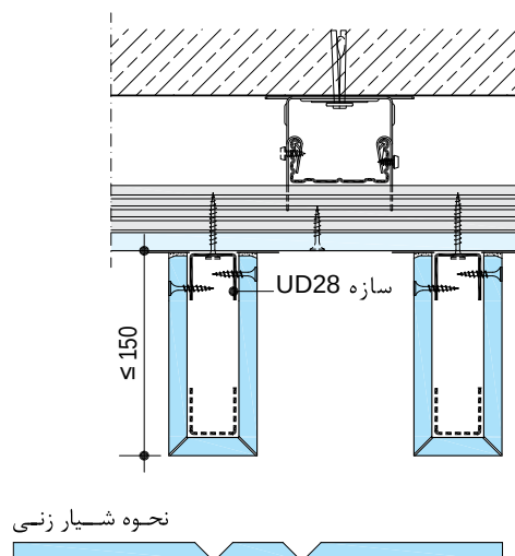
سقف کاذب با تیغه‌های قائم
