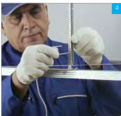
۵ اتصال چنگک به آویز و رگلاژ سقف توسط پین
