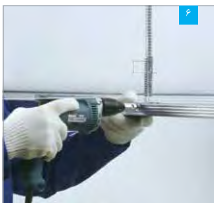
۶ اتصال سازه باربر به چنگک توسط پیچ LN
