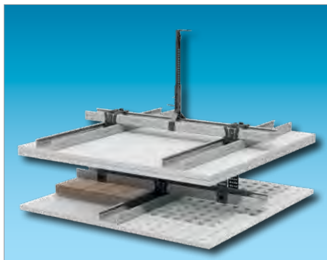
مثال: سقف کاذب یکپارچه D112 فاقد کد حریق زیر سقف کاذب یکپارچه D112 دارای کد حریق از پایین سقف
