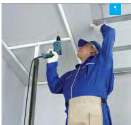
۹ اتصال پنل به زیرسازی توسط پیچ
