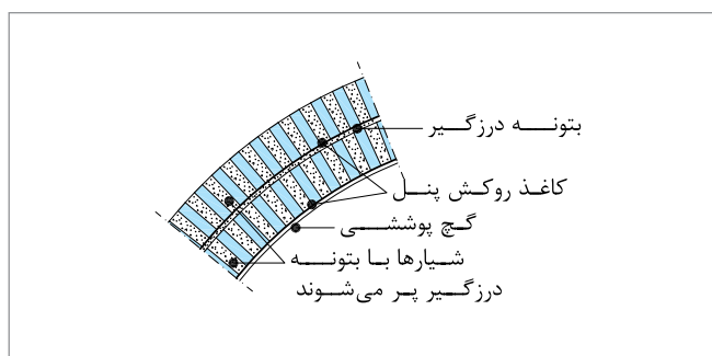
پوشش کاری دو لایه
