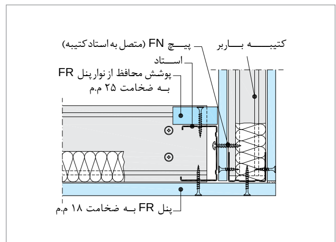
اتصال سقف کاذب خود ایستا به کتیبه باربر
