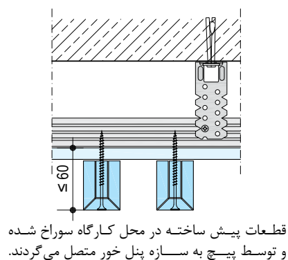
سقف کاذب با تیغه‌های قائم
