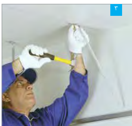
۳ اتصال آویز به سقف اصلی
