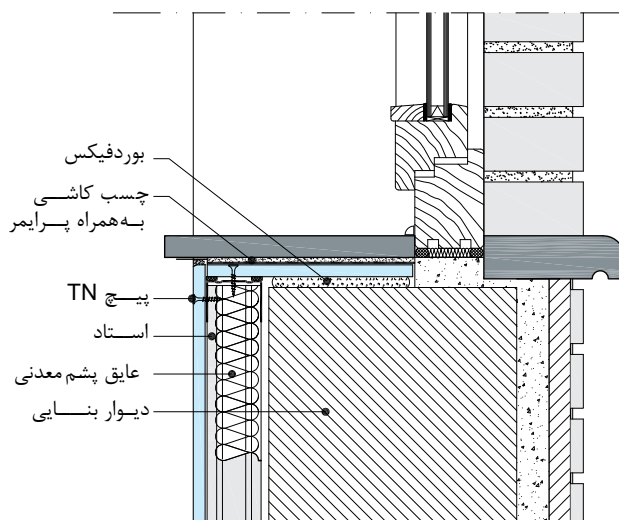
پوشش کاری دور پنجره و جزئیات نصب سنگ کف پنجره W625.ir
