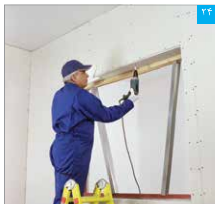
اتصال پنل نواری به رانر قاب بندی فوقانی
