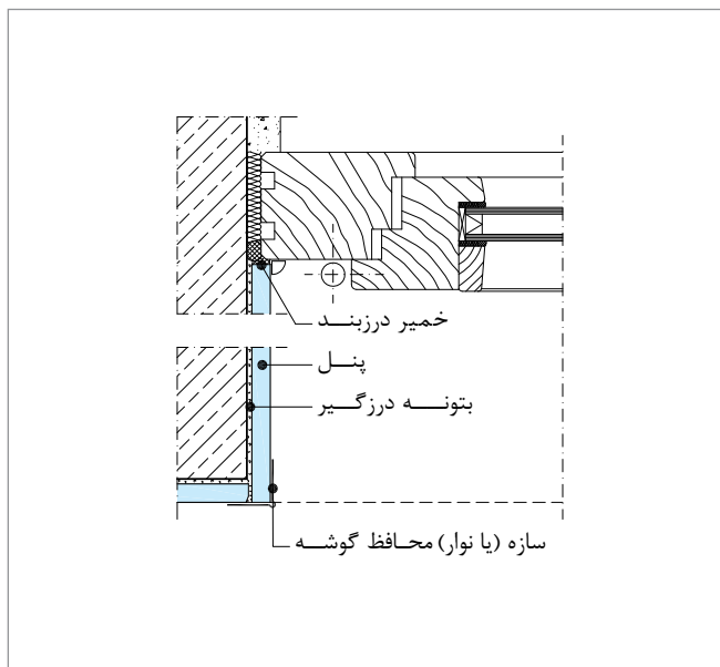
پوشش‌کاری دور پنجره
