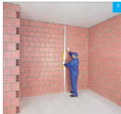
مشخص کردن محل اجرای چانه‌های چسب گچی پنل (بوردفیکس) بر روی دیوار زمینه
