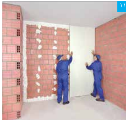
استقرار پنل بر روی دیوار زمینه
