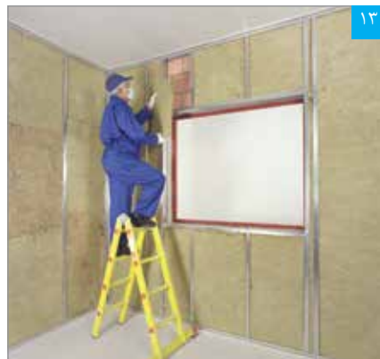
اجرای عایق پشم معدنی
