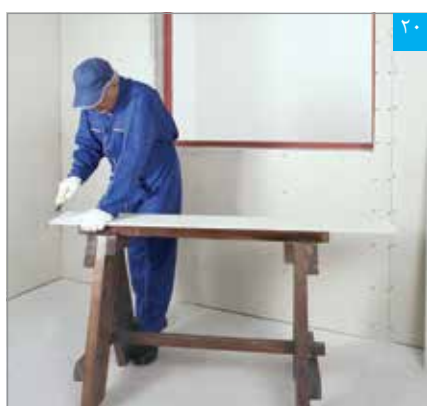
برش پنل نواری (برای پوشش کاری ناحیه داخلی دور بازشوی پنجره)
