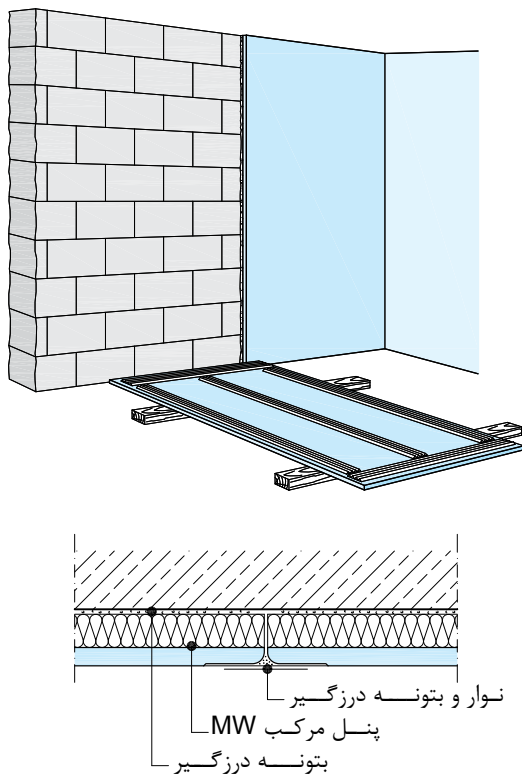
لایه نازک بتونه درزگیر
